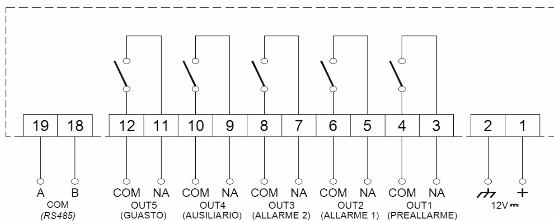
Рис. 2 Схема подключения
